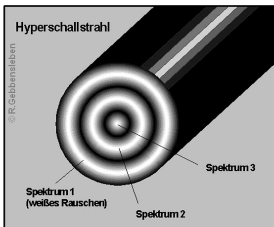
Bild 3: Die Struktur der Hyperschallstrahlen
